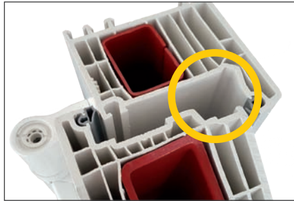
Wandstärke bis 3,5 mm für optimale Stabilität
