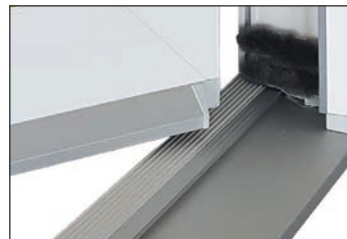
Wetterschenkel seitlich verschlossen / Bodenschwelle thermisch getrennt
